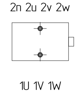
Рис.1. Схема исполнения вводов.
